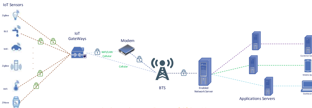
شکل ۱ جایگاه گیت‌وی در اکوسیستم اینترنت اشیا
