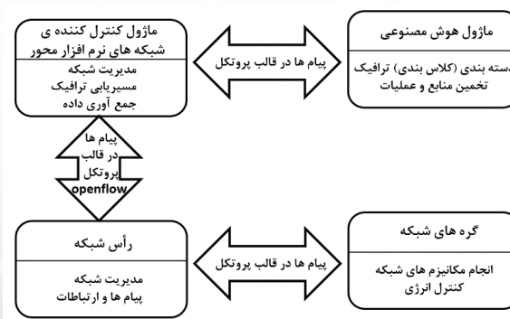
شکل ۱- نحوه اتصال ماژول هوش مصنوعی به پیکره شبکه‌های نرم‌افزار
